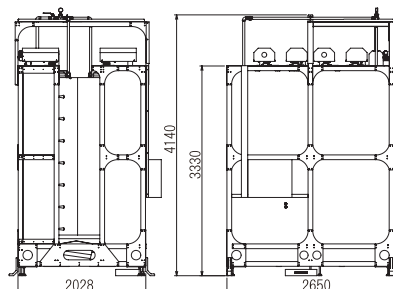
机械式样
